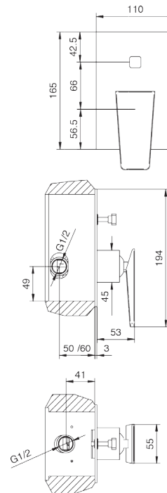
UP-Körper Art.Nr.: 45.749.12.00 concealed body ref.no.: 45.749.12.00
